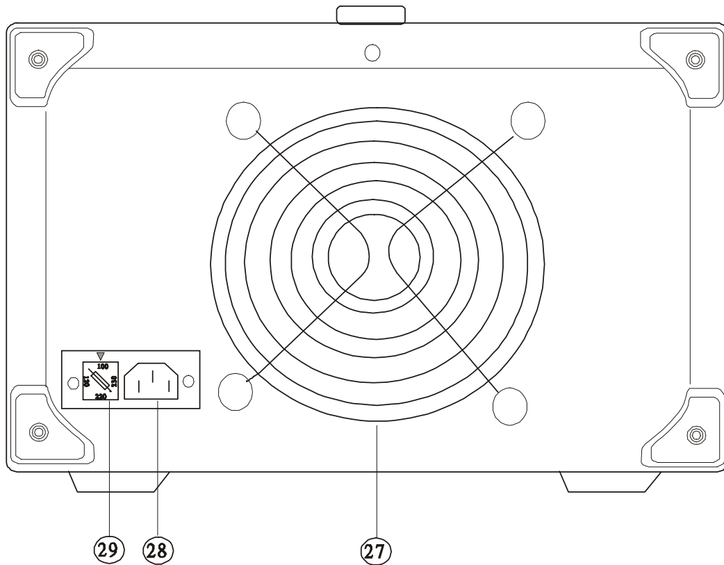
9303D，9603D，9306D 背板圖
