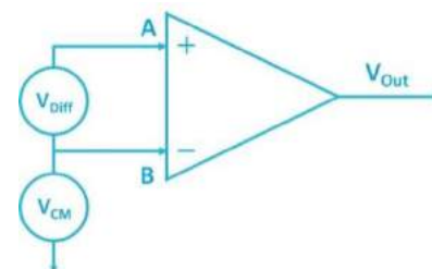
圖 2：差動式量測
