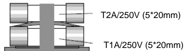
圖 2-2 保險絲座
