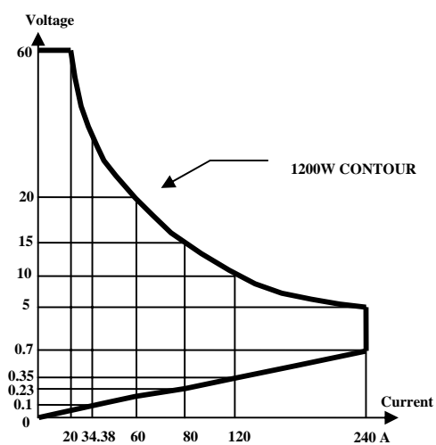
圖 1-3 3352F 高功率電子負載功率曲線圖
