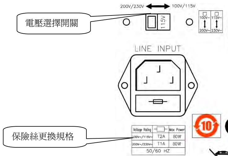
圖 2-1 電源設定圖
