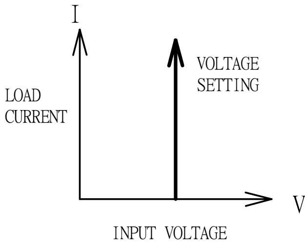
圖 1-9 固定電壓模式特性圖
