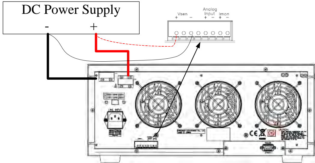
圖 3-3 典型 3350F高功率電子負載連接方式
